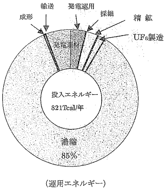
第3図 ガス拡散法ウラン濃縮による原子力発電の投入エネルギーの内訳 3)
