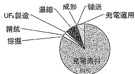
第4図 遠心ウラン濃縮による原子力発電の投入エネルギー内訳
