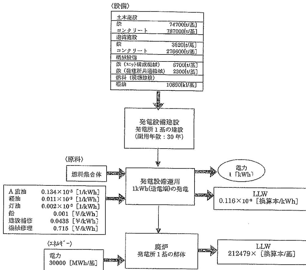
第7図 原子力発電所の入力エネルギー 6)
